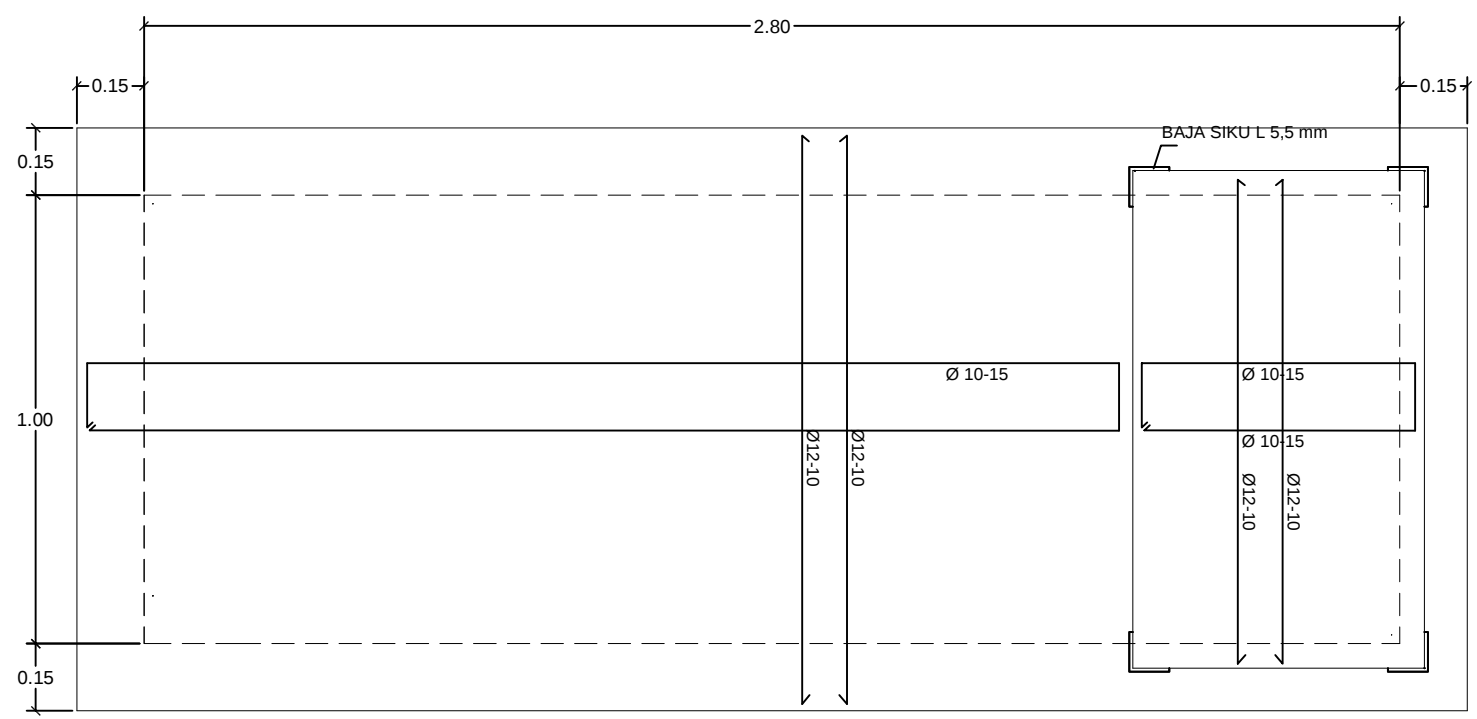
PEMBESIAN BOX VALVE SKALA 1 : 15
